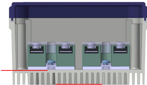
Exemple de montage de relais statiques sur un boîtier aluminium Ultimheat. (Graisse thermique en rouge)
